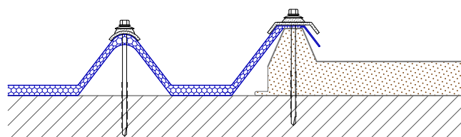
Abbinamento laterale a pannelli metallici
