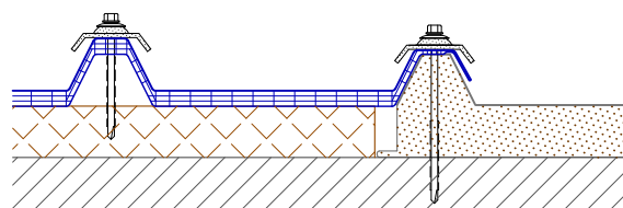
Abbinamento laterale a pannelli metallici
